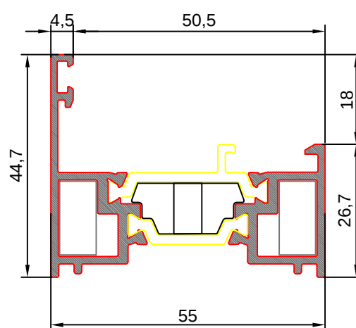
anta centrale ES 583940 g/m 1059
