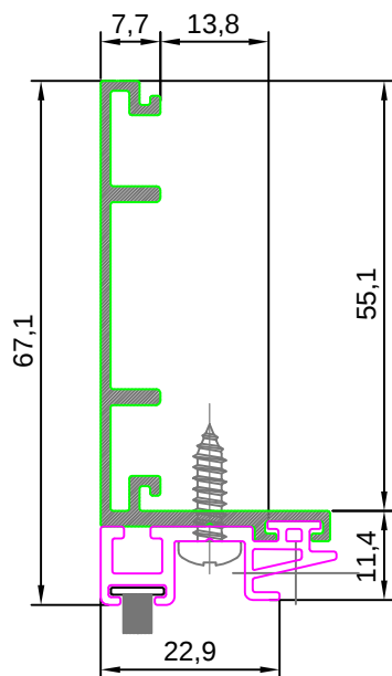
Profilo centrale ES 5807 g/m 492
