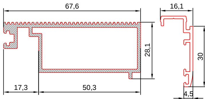
Profilo di transito ES 5818 g/m 931
