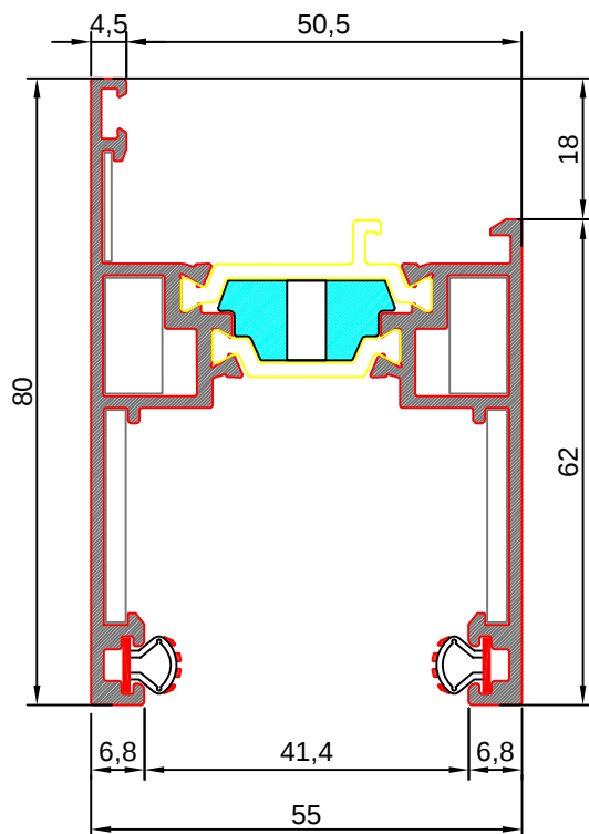
Anta ES 580203 g/m 1518
