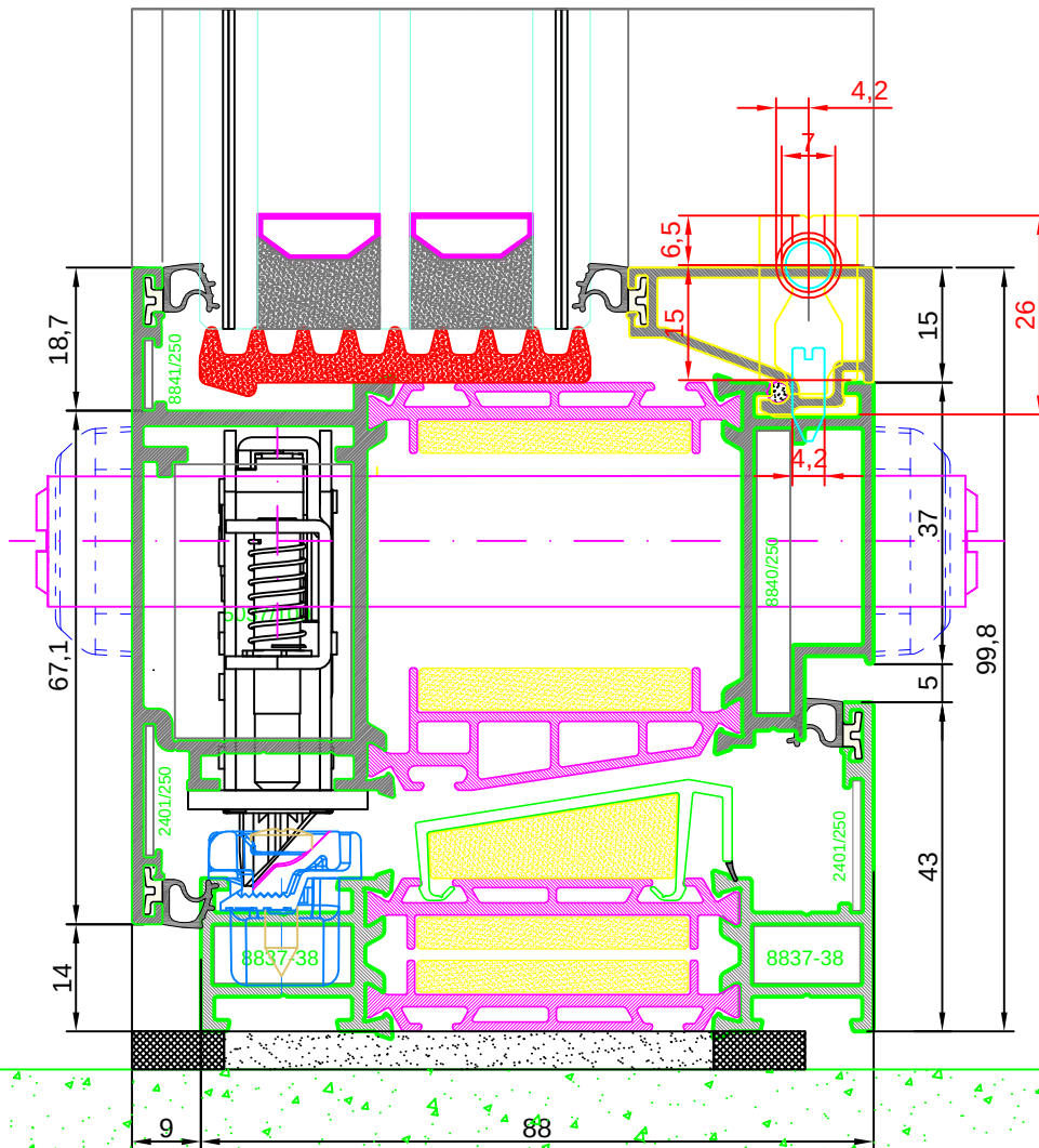
Traverso anta apertura esterna
